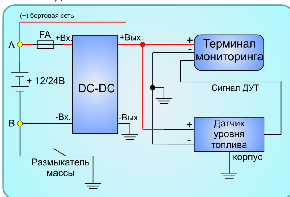
Рисунок 7 – Схема подключения с дополнительным DC-DC преобразователем
