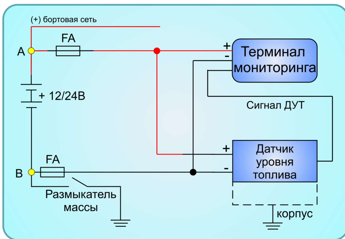
Рисунок 6 – Схема подключения после размыкателя массы
