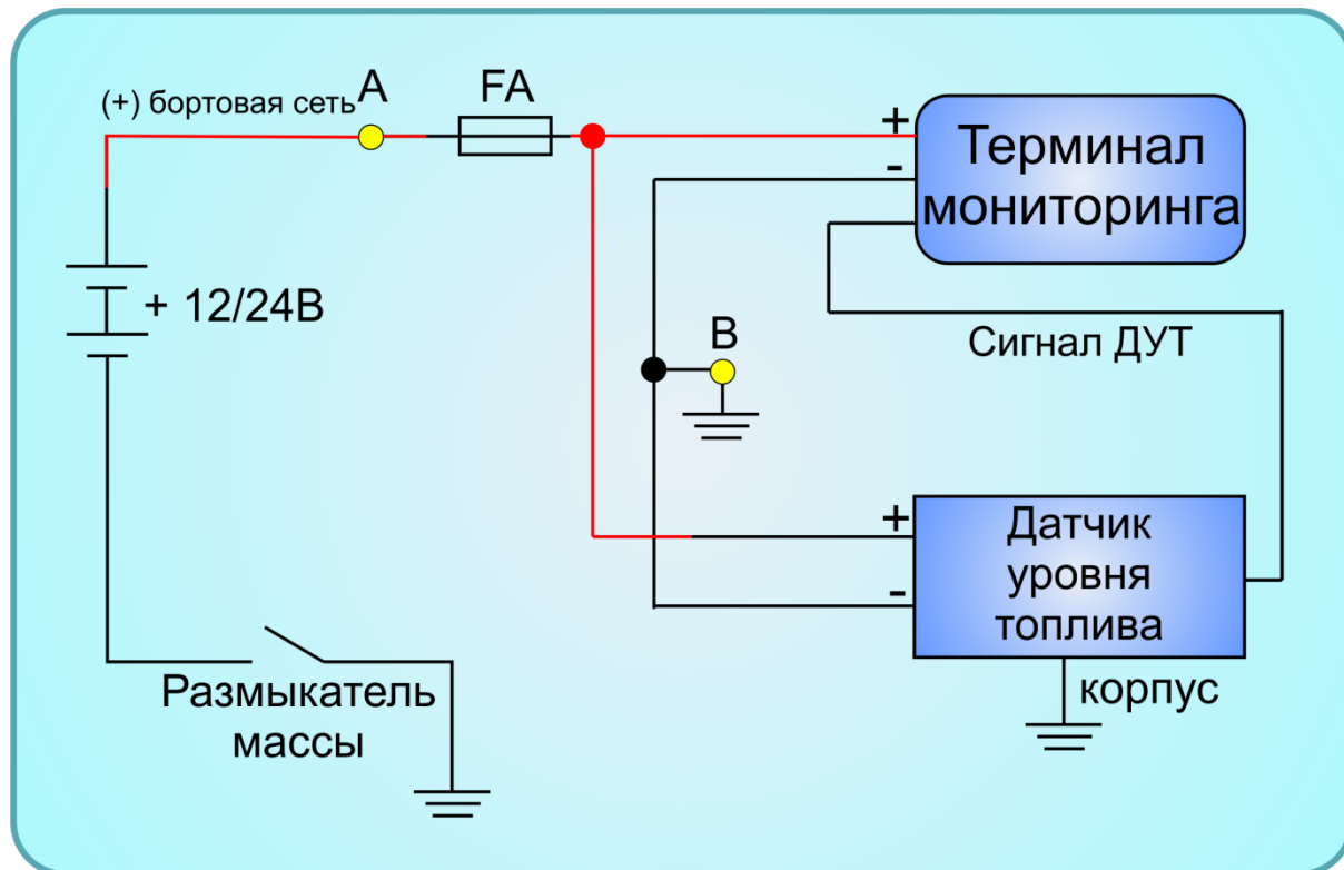
Рисунок 5 – Схема подключения до размыкателя массы
