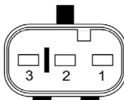
Рисунок 4 – Разъем ДУТ.А
